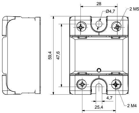
GN+ Vorderansicht
