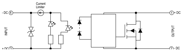
Control DC serie GNAD
