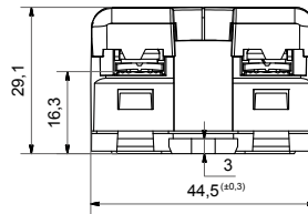
Vista lateral GNAD
