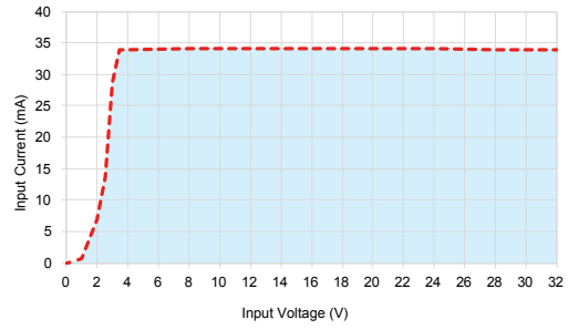
Corriente de entrada frente a voltaje de entrada Entradas de DC reguladas estándar
