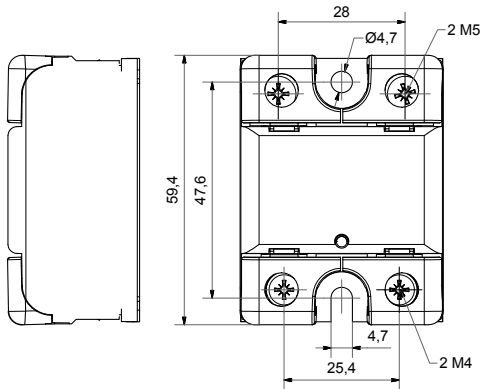
Vista frontal GNAD
