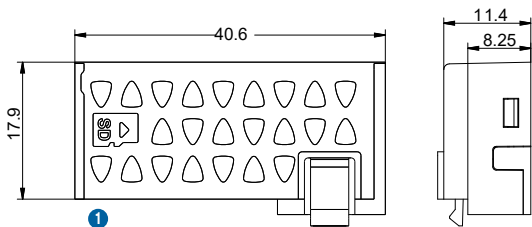
1 Emplacement pour carte SD
