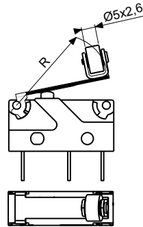
170EL à galet latéral
