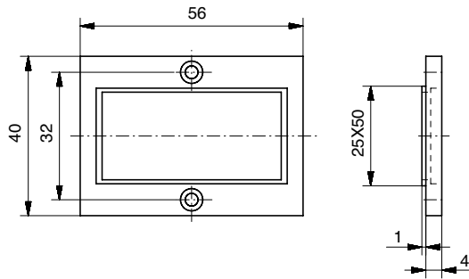
26546843 - Adattatore per foro 50 x 25 mm - Fissato con viti
