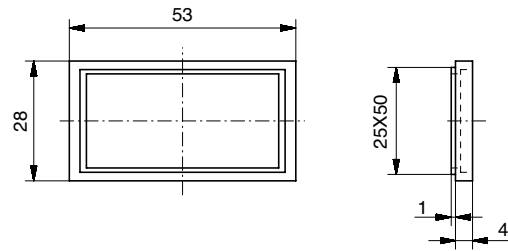
26546844 - Adattatore per foro 50 x 25 mm - Fissato con clip
